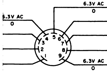
RF AMPLIFIER V202A/V202B 12AT7
