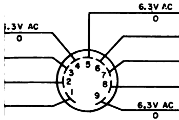
DETECTOR V203A/V203B 12AT7
