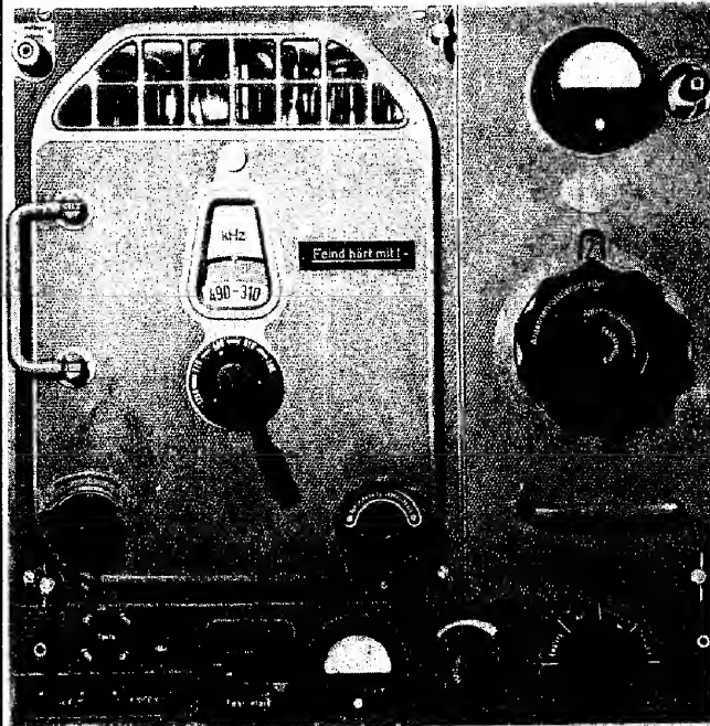
100 W. S. (GROUND TRANSMITTER)
