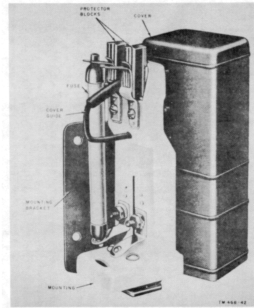
Figure 51. Protector AR-6A (Cookeco. No. 0-9).
