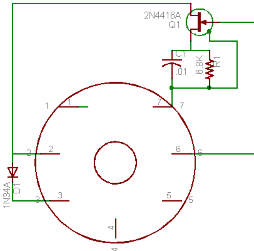
1L4 Module RT77/GRC-9 V1 RF Amplifier
